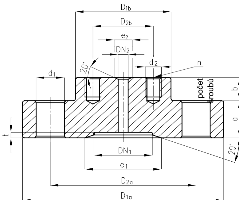
Přechod přírubový DN58/DN10 z oceli 12020 podle N16.81
